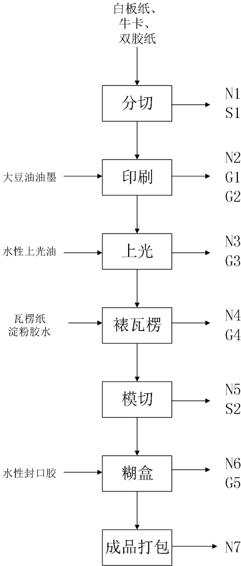
图 2-2 各类环保型彩色包装生产工艺流程图 (注：Gn：废气污染物；Sn：固体废弃物；N：噪声)
