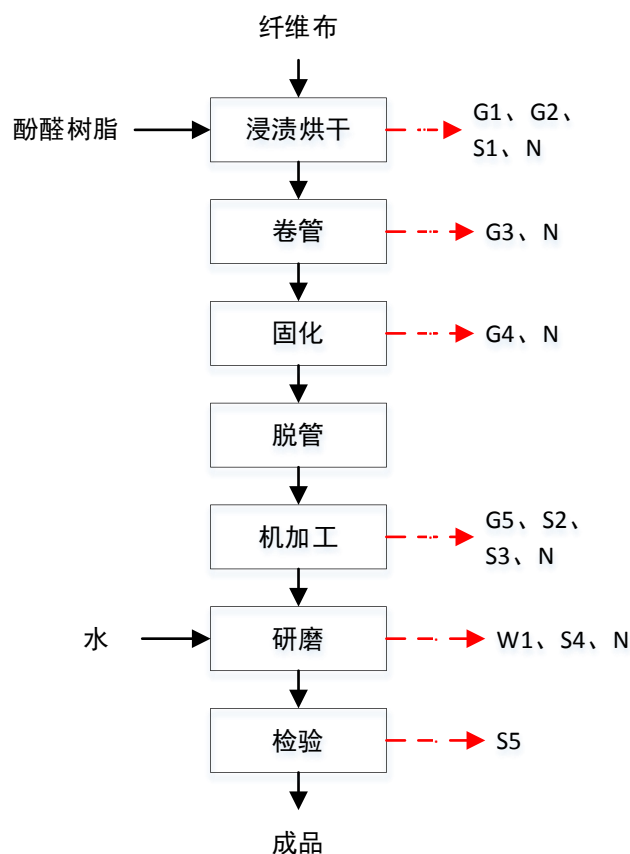
图 2-2 支撑环工艺流程图
