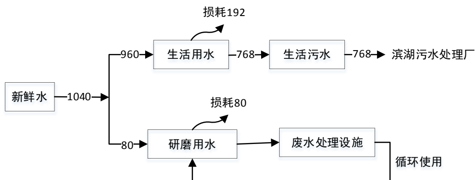
图 2-1 验收项目水平衡图
