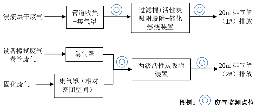
图 3-2 有组织废气处理流程图及监测点位
