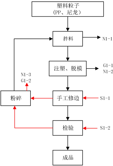
图 2-2 塑料制品生产工艺流程图 (注：Gn：废气污染物；Sn：固体废弃物；N：噪声)
