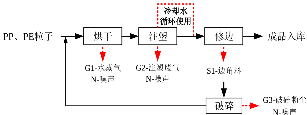
图 2-1 塑料制品工艺流程图
