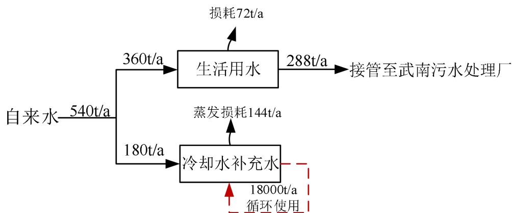
图 4-2 水平衡图
